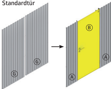
Standardtür
